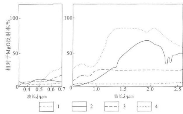
图 2 含铁矿物的波谱曲线( 据文献[5])
