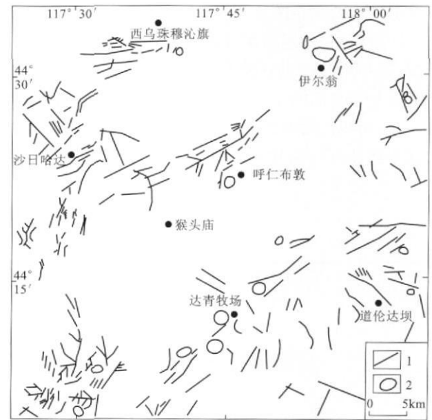
图 4 ETM+ 遥感影像构造解译图
