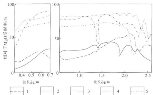
图 3 含羟基(OH - )与碳酸根矿物的波谱曲线(据文献[ 5])
