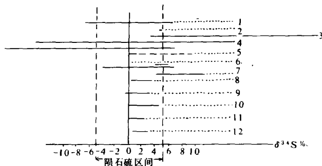
1. 浙东某矿区 2. 美国特克汤 3. 澳大利亚芒特艾沙 4. 德国兰姆乐斯别尔格 5. 澳大利亚布尔肯希尔 6. 日本柯罗科 7. 安徽新桥矿区 8. 加拿大魁北克 9. 苏联高加索 10. 苏联乌拉尔 11. 瑞典弗兰恒 12. 瑞典布利登
