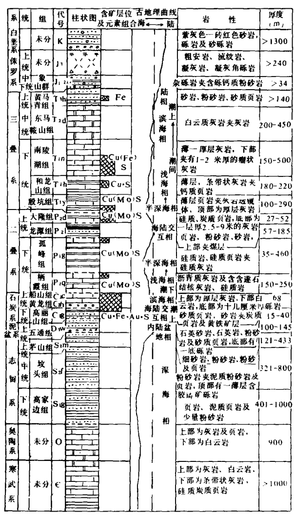
图3 铜陵地区地层综合柱状图
