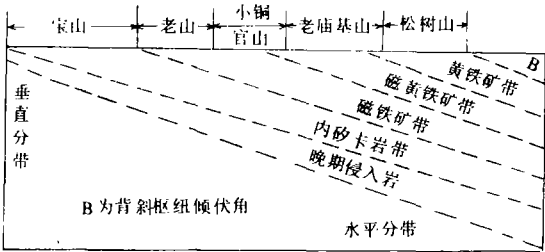
图 11 铜官山矿床层状矿体改造分带示意图
