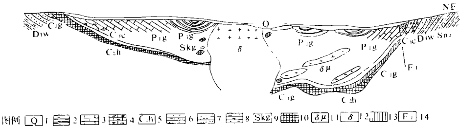
1. 现代堆积 2. 孤峰组 3. 栖霞组 4. 船山组 5. 黄龙组 6. 高骊山组 7. 五通组 8. 寨山组 9. 砂卡岩 10. 矿层 11. 闪长玢岩 12. 石英闪长岩 13. 高岭土化 14. 断层
