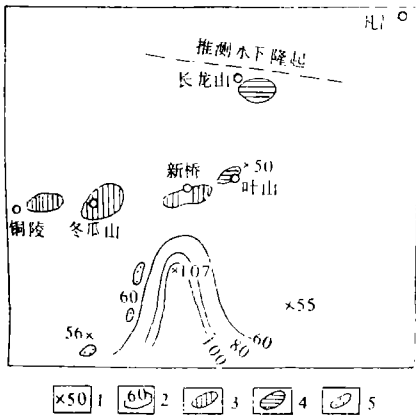
1. 剖面地点及地层厚度 2. 等厚线 3. 铜硫铁矿床 4. 铁矿床 5. 深部为硫铁矿
