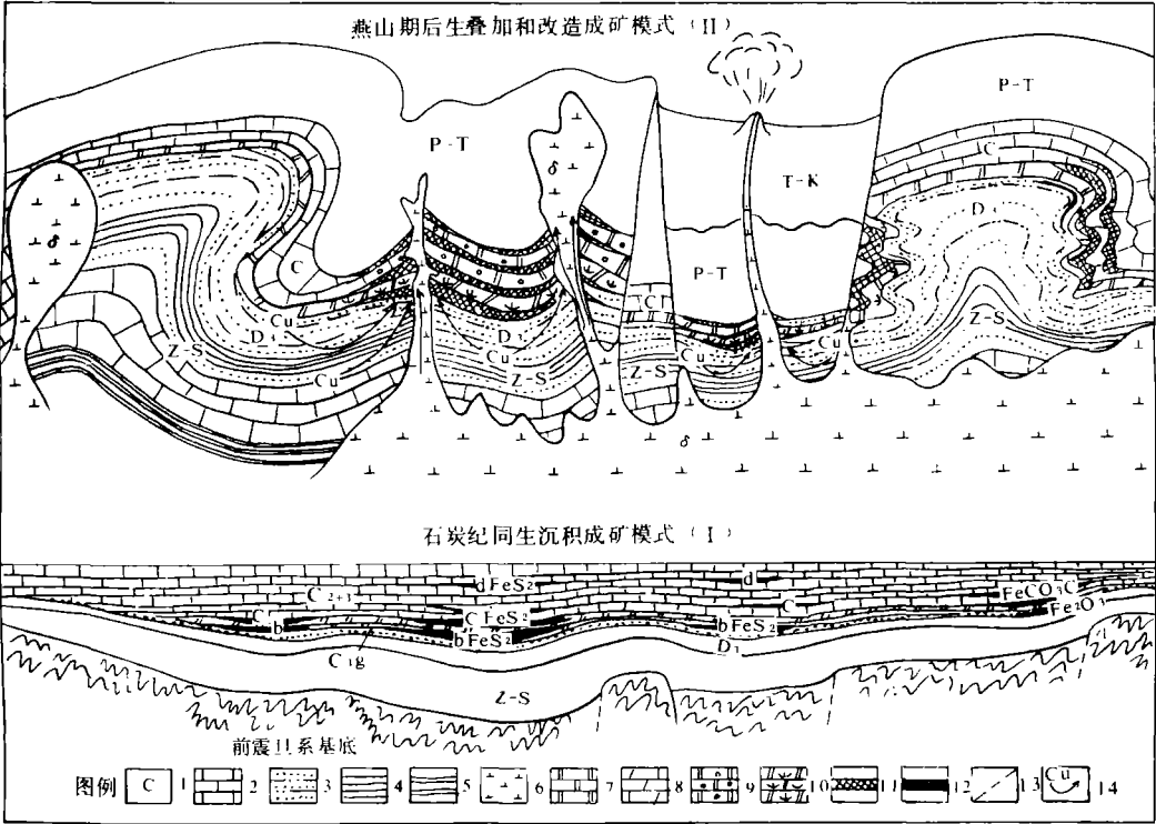
1.组合 2.灰岩 3.砂岩 4.页岩 5.硅质岩 6.闪长岩类侵入岩 7.大理岩 8.白云质大理岩 9.矽卡岩 10.蛇纹石化白云岩 11.改造叠加矿层 12.沉积矿层 13.断层 14.矿液迁移方向
