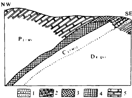
1. 石英岩 2. 角闪岩 3. 铁帽 4. 铜矿体 5. 大理岩
