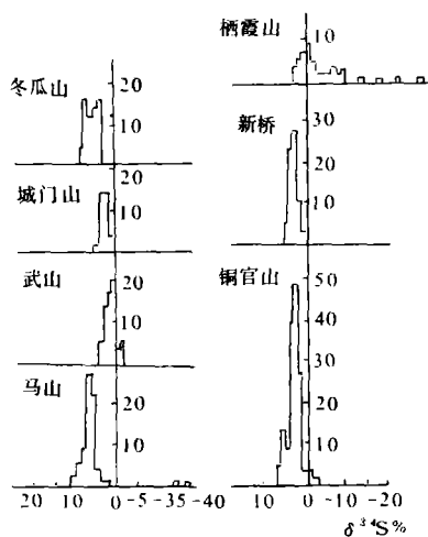
图 12 长江中、下游含铜硫化物矿床硫同位素组成直方图
