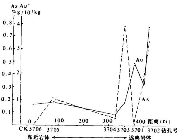
图 11 马山矿区第 37 线各钻孔金、砷平均含量变化图 (横坐标为各钻孔见矿部位的水平距离)
