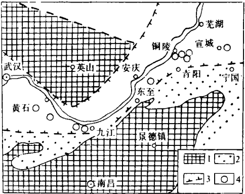
1. 前寒武纪古陆 2. 加里东边缘冒地槽 3. 断裂拗陷带边界 4. 含铜硫化物矿床
